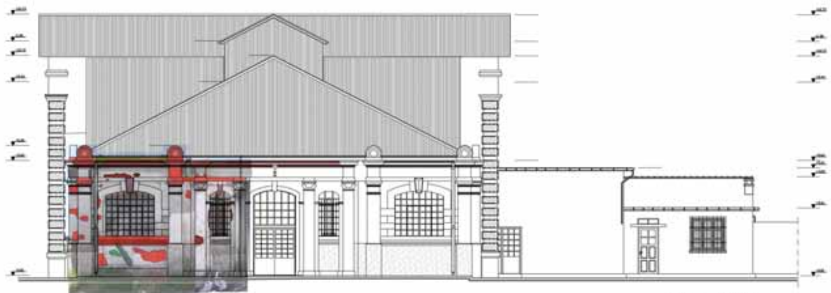
ΟΡΘΗ ΑΝΑΤΟΛΙΚΗ
