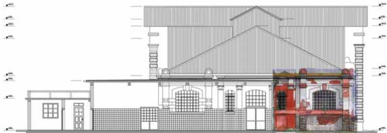
ΟΡΘΗ ΑΥΤΙΚΗ
